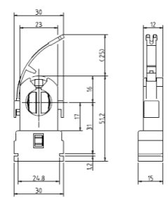
脱着防止ソケット写真及び完成図
