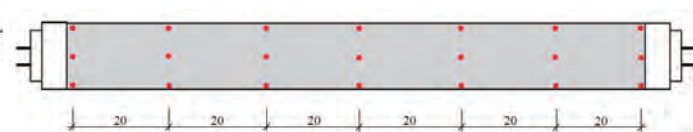
直管型ランプの明るさ分布測定ポイントのイメージ図 単位：cd/m²
