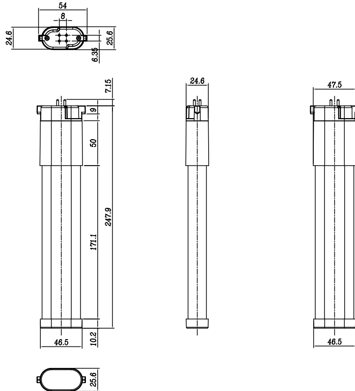
外形寸法(mm)
