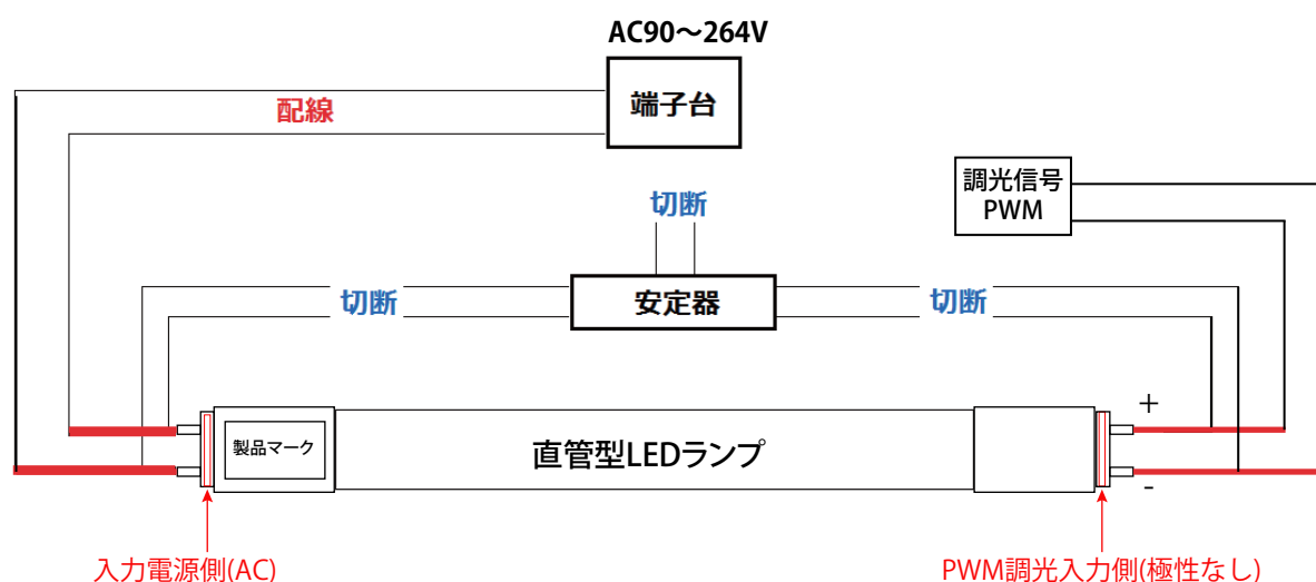
直管型LEDランプ・器具内配線図(標準規格)
