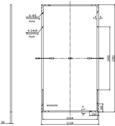
背面図 (mm)
